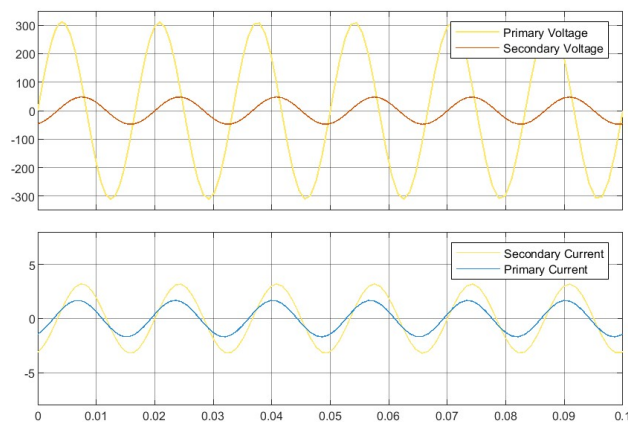
Рис. 10. Графики напряжения и тока на обмотках трансформатора
