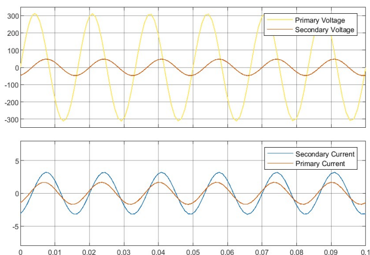
Рис. 17. Графики напряжения и тока на обмотках трансформатора при изменении индуктивности цепи намагничивания
