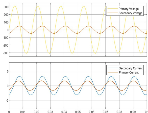
Рис. 11. Графики напряжения и тока на обмотках трансформатора при изменении номинальной мощности
